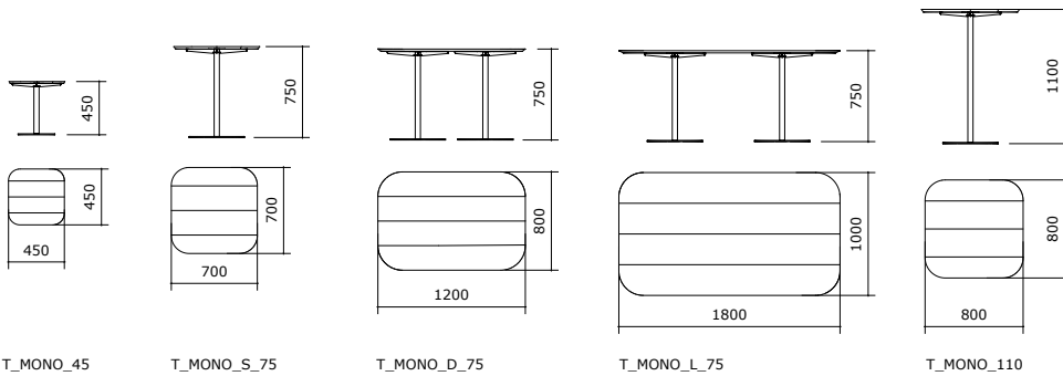
MONO™ TABLE
